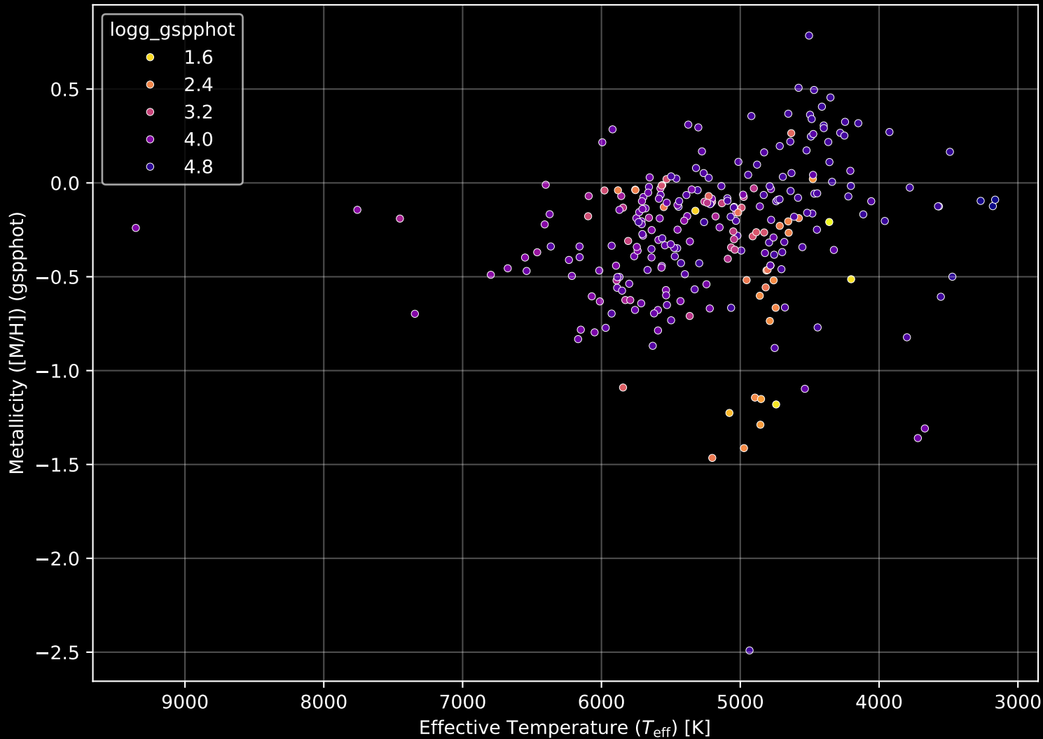
APOGEE DR17 Field: [024+64_btx] Stellar Population Parameters (n= 265)
